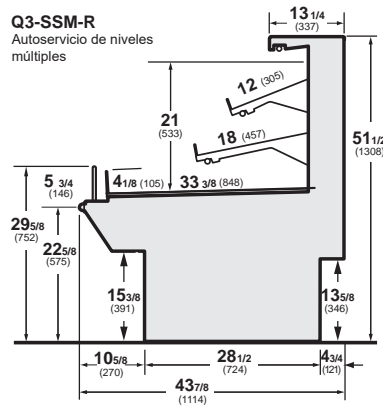
Q2/Q3-SSM-R Autoservicio de niveles múltiples
