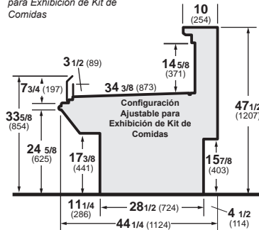
Q2-SSM-R Autoservicio de niveles múltiples Configuración Ajustable para Exhibición de Kit de Comidas
