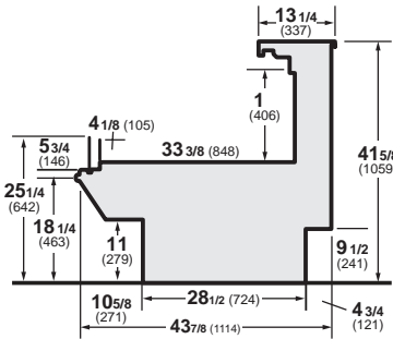
Q3-SSM-R Autoservicio de niveles múltiples
