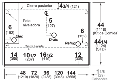
Q2/Q3-SSM-R Autoservicio de niveles múltiples
